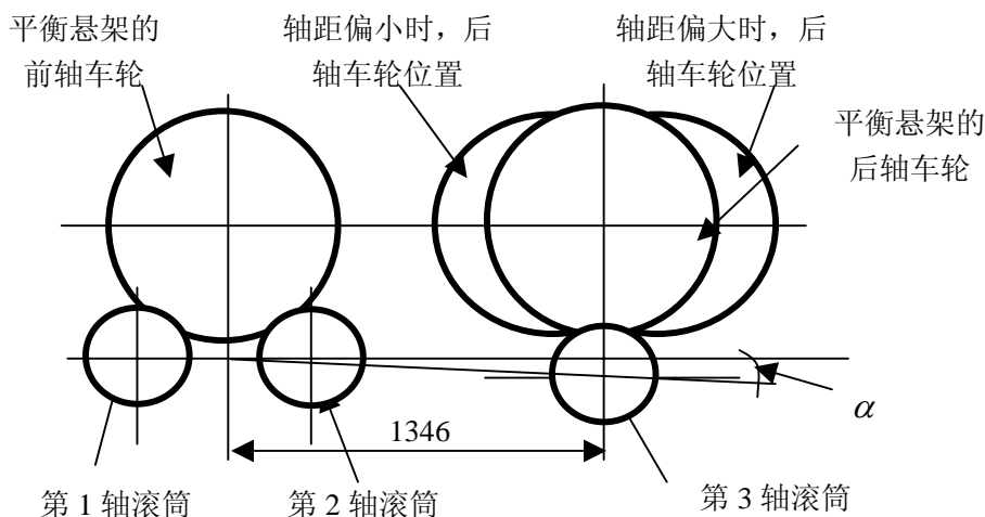
图 1 3 轴 6 滚筒的底盘测功机滚筒布置示意图
