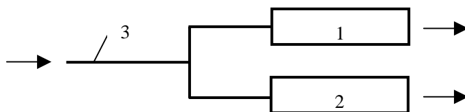
图 2 不透光烟度计的有效长度 L 检测装置示意图
